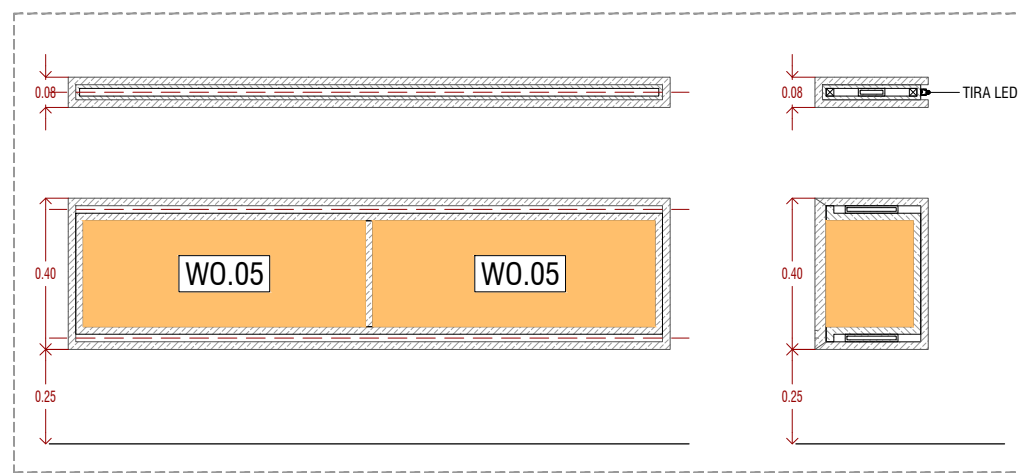
SECCIÓN LONGITUDINAL
