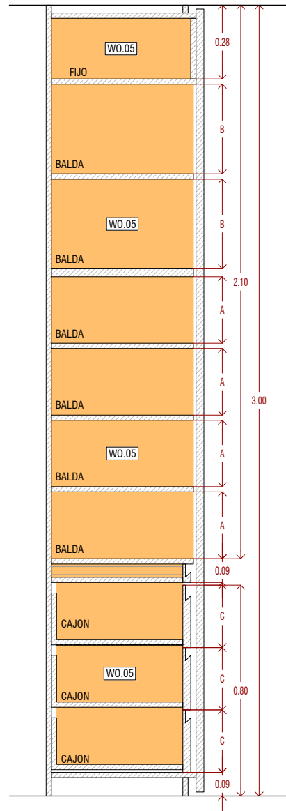
SECCIÓN 04
