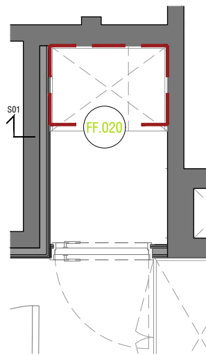
PLANTA
