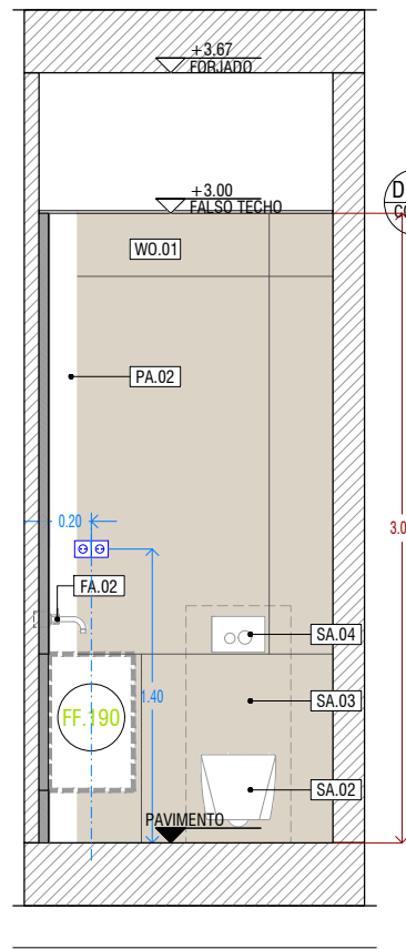
SECCION 02
