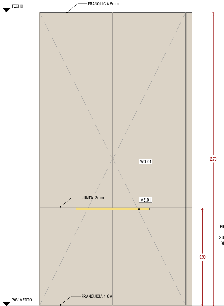
ALZADO
