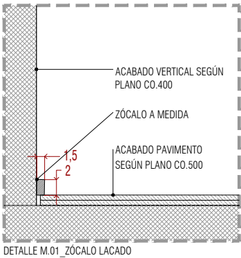
DETALLE M.01 _ZÓCALO LACADO
