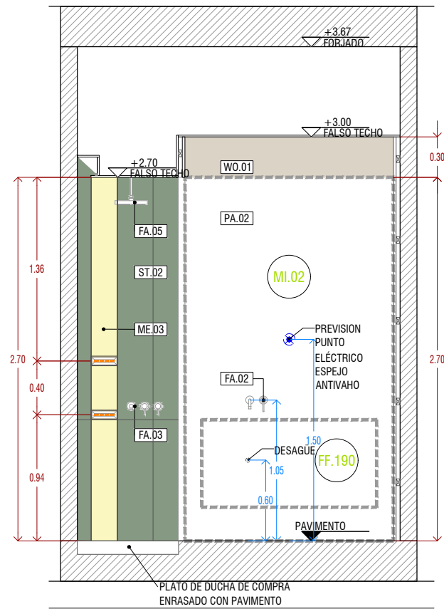
SECCION 01
