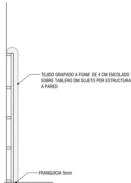
SECCIÓN
