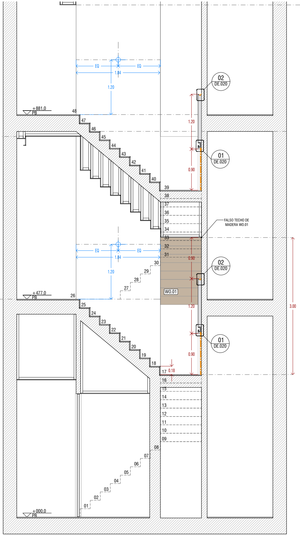
SECCIÓN 02
