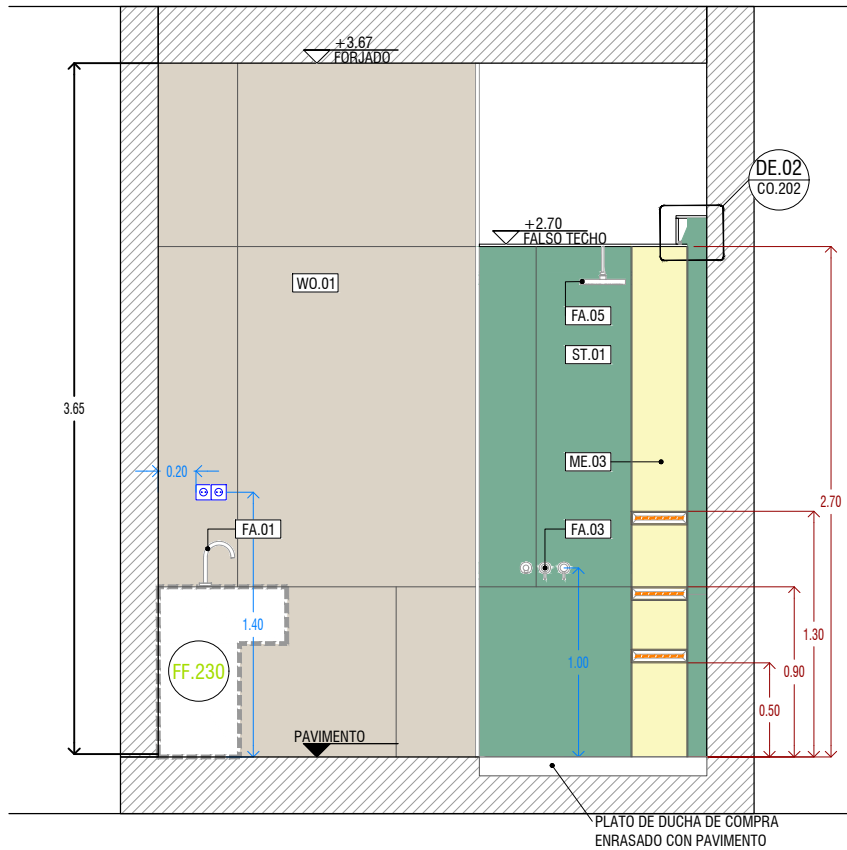
SECCION 03
