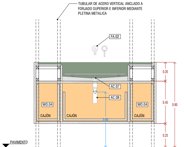
SECCIÓN 01
