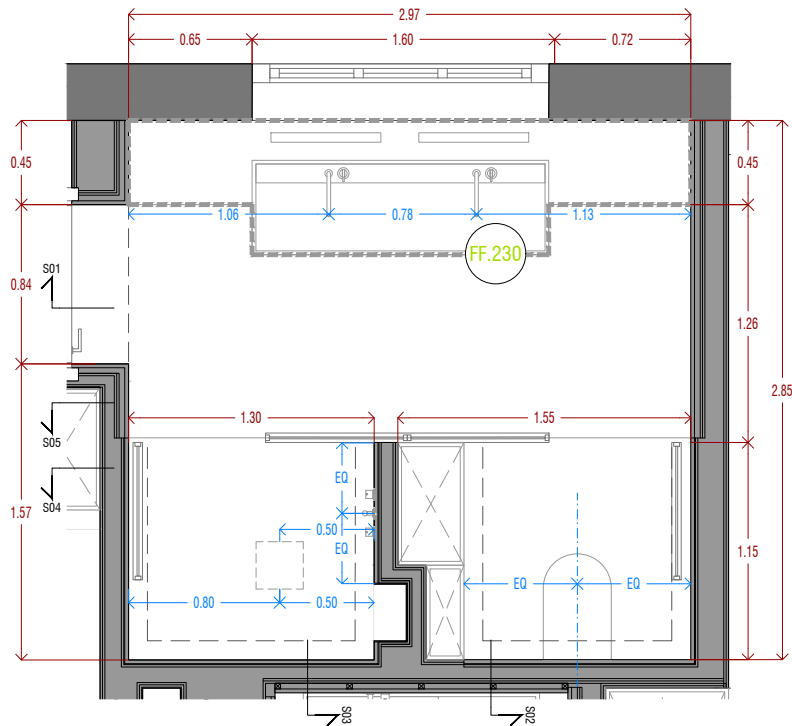
PLANTA
