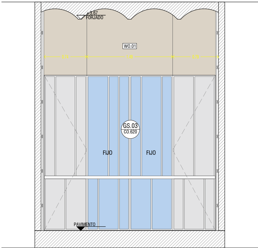
SECCION 05
