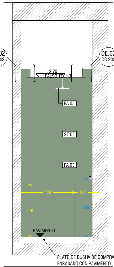
SECCION 03
