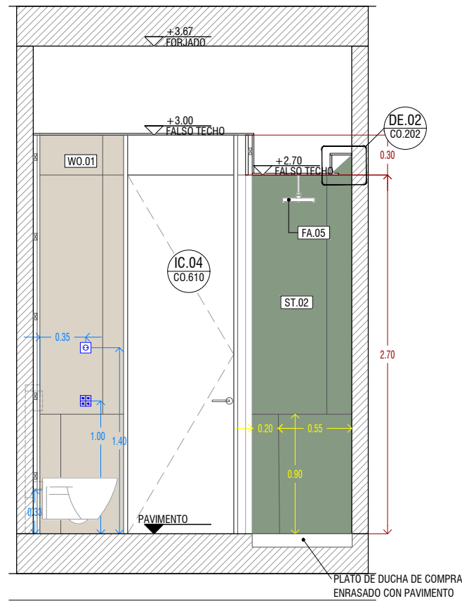
SECCION 04
