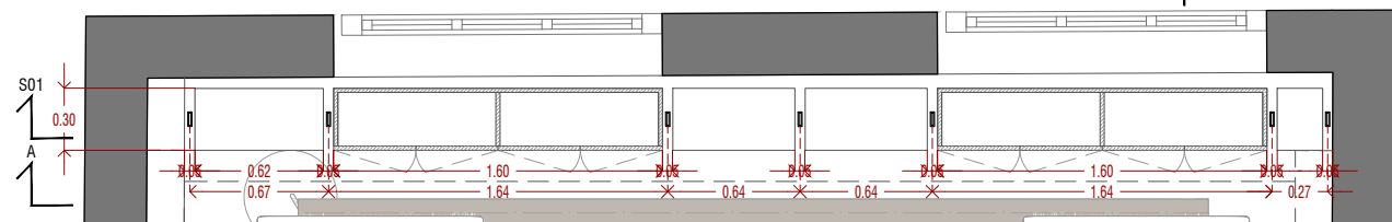
PLANTA
