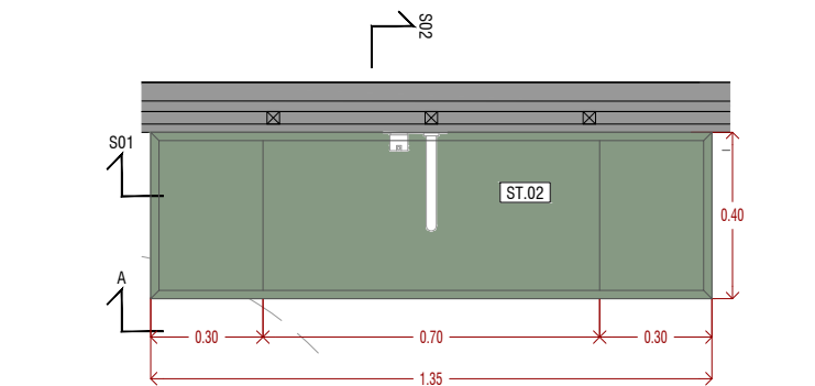
PLANTA
