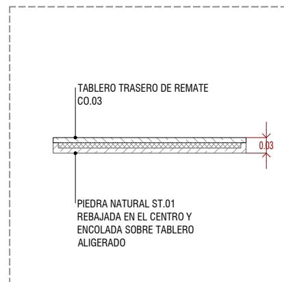
DETALLE D.01 PUERTA DE ARMARIOS
