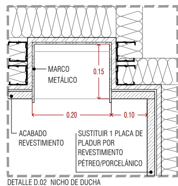
DETALLE D.02 _NICHOS DE DUCHA
