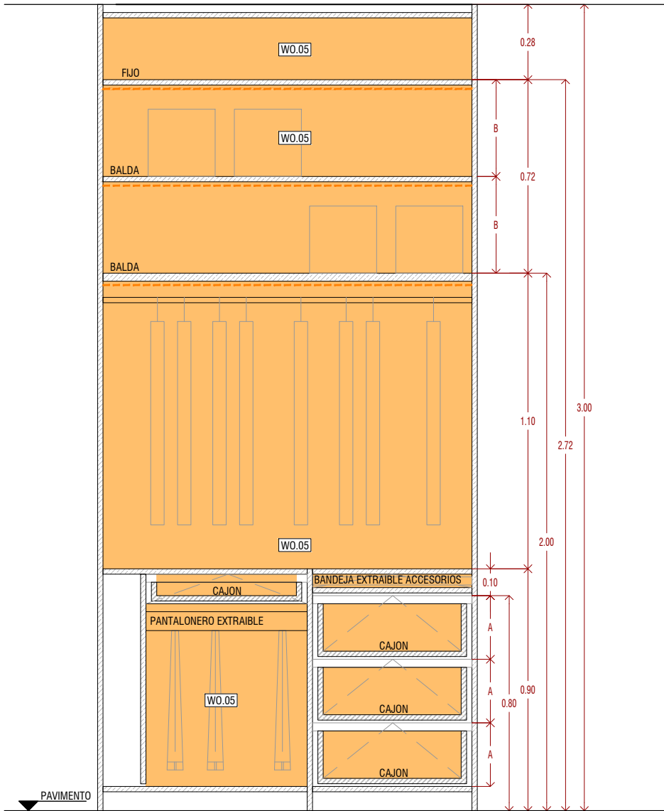
SECCIÓN 01
