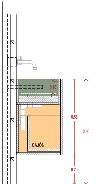
SECCIÓN 02
