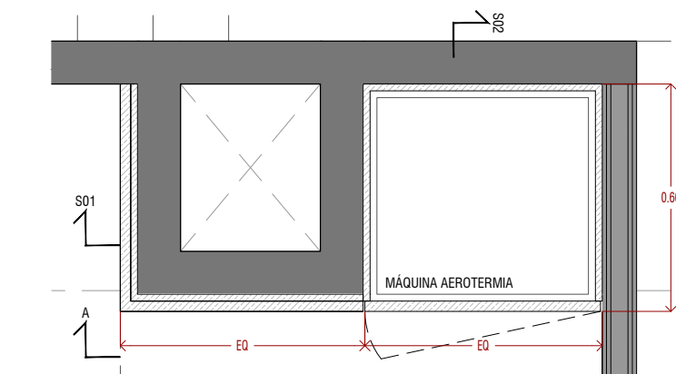
PLANTA
