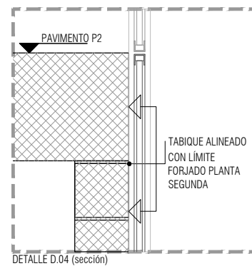
DETALLE D.04 (sección)
