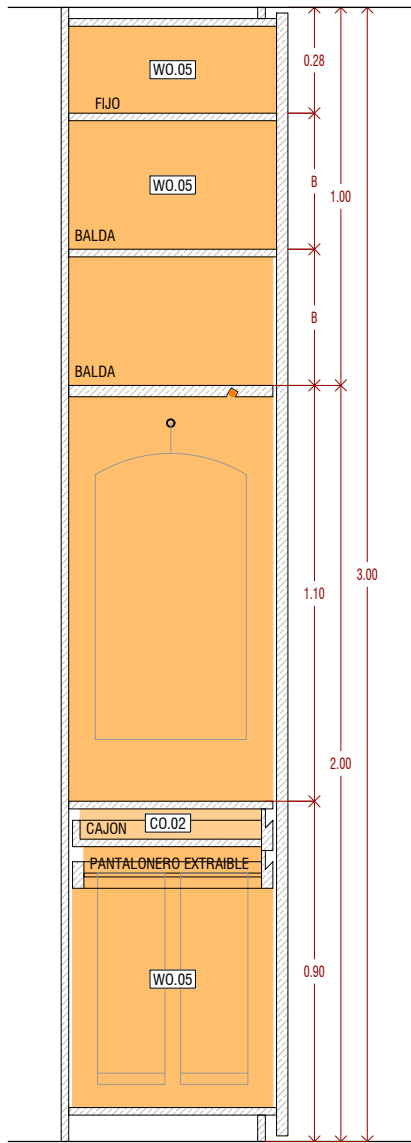
SECCIÓN 02
