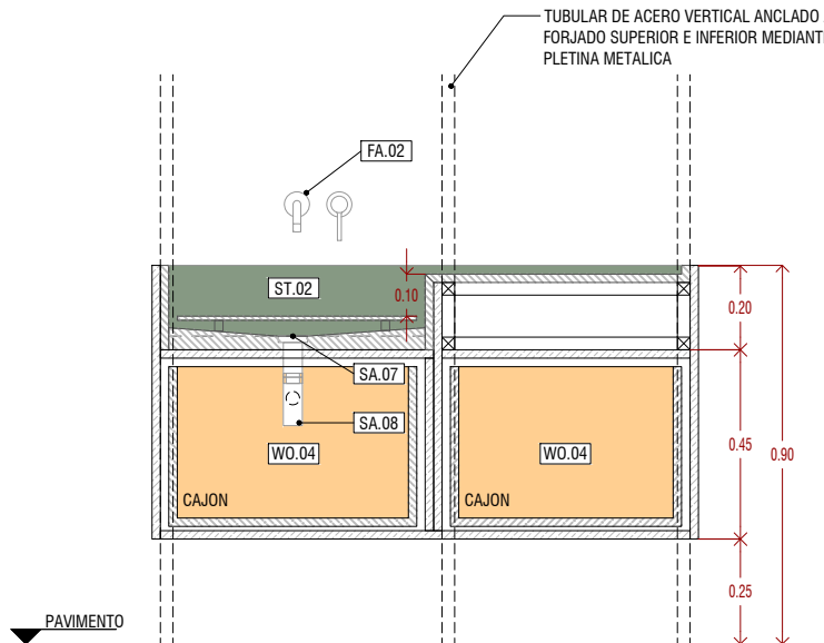
SECCIÓN 01
