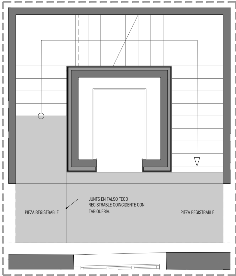
DESPIECE DE TECHO REGISTRABLE. RECIBIDOR P1
