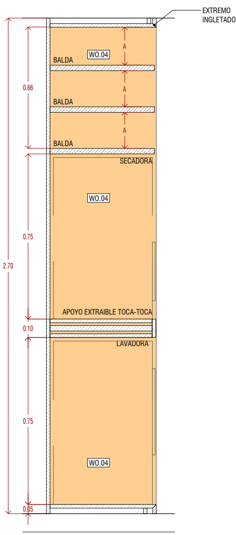
SECCION 01
