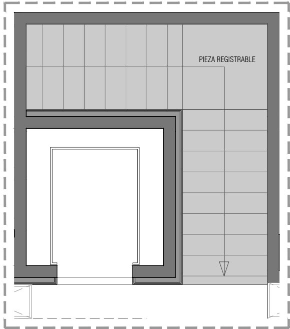
DESPIECE DE TECHO REGISTRABLE. ESCALERA P2
