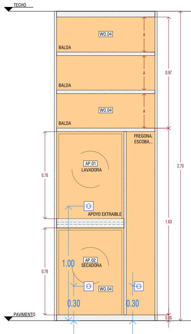
ALZADO
