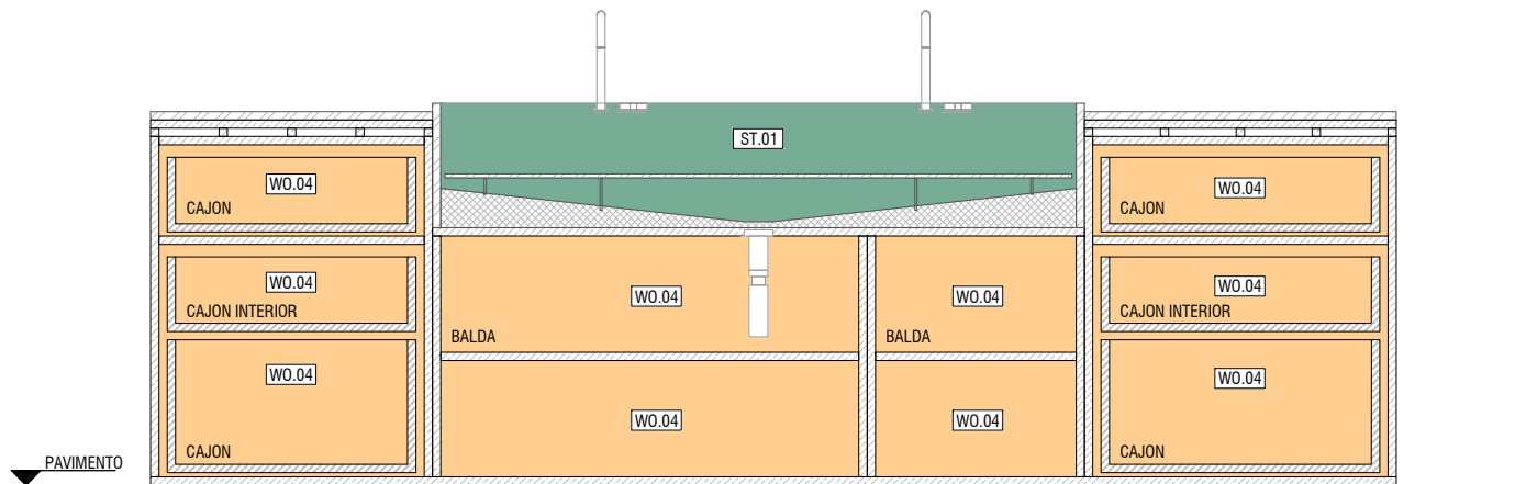
SECCIÓN LONGITUDINAL
