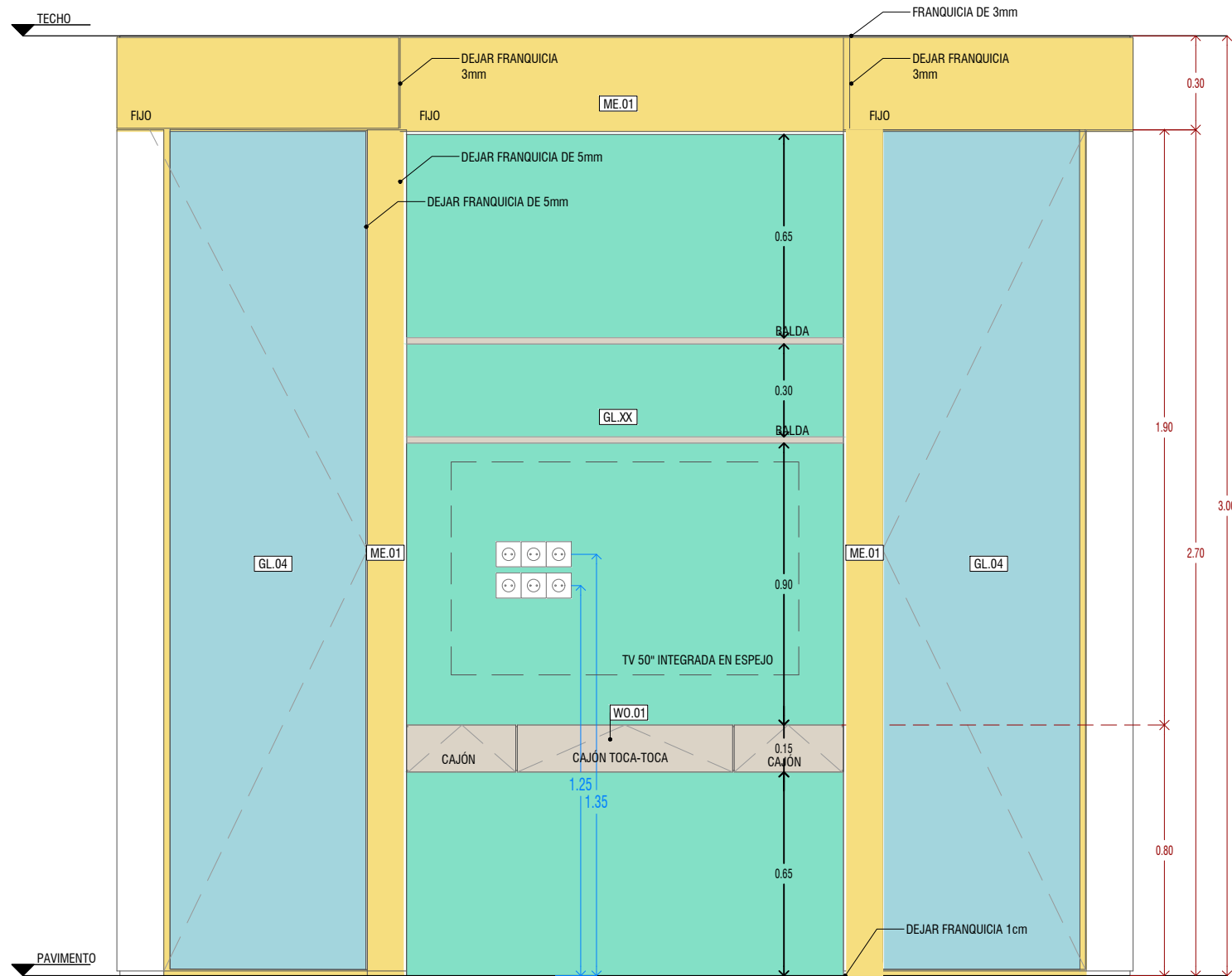
ALZADO
