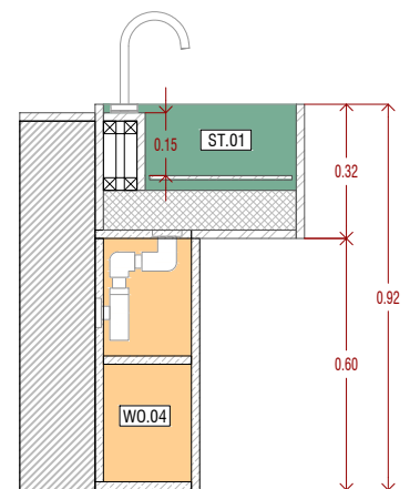
SECCIÓN TRANSVERSAL
