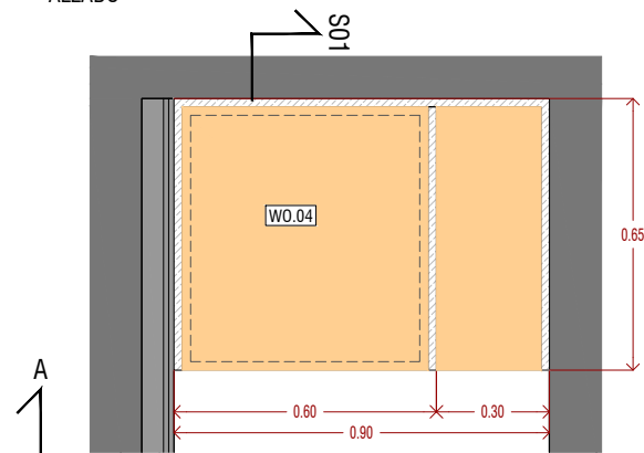
ALZADO
