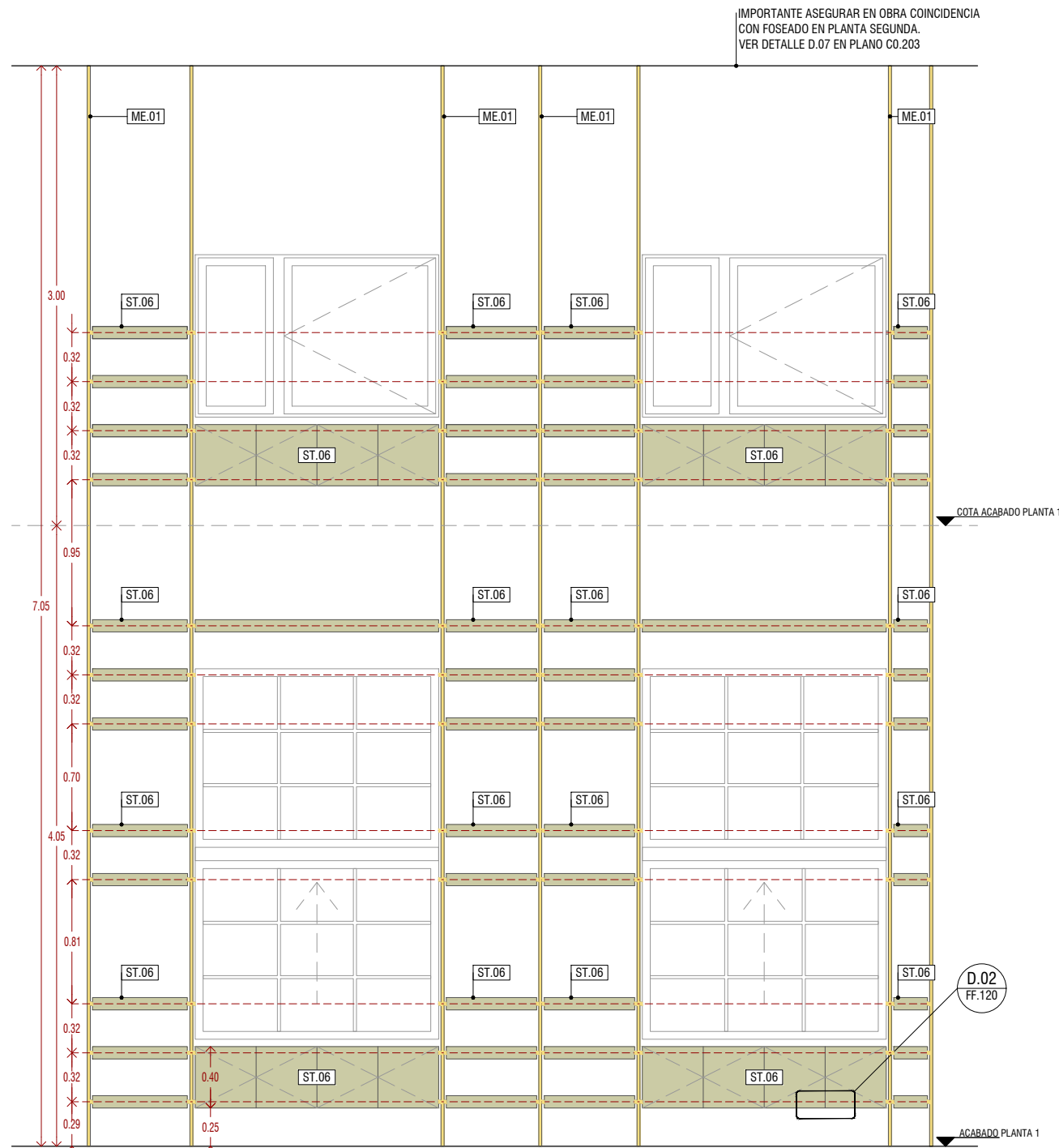
ALZADO
