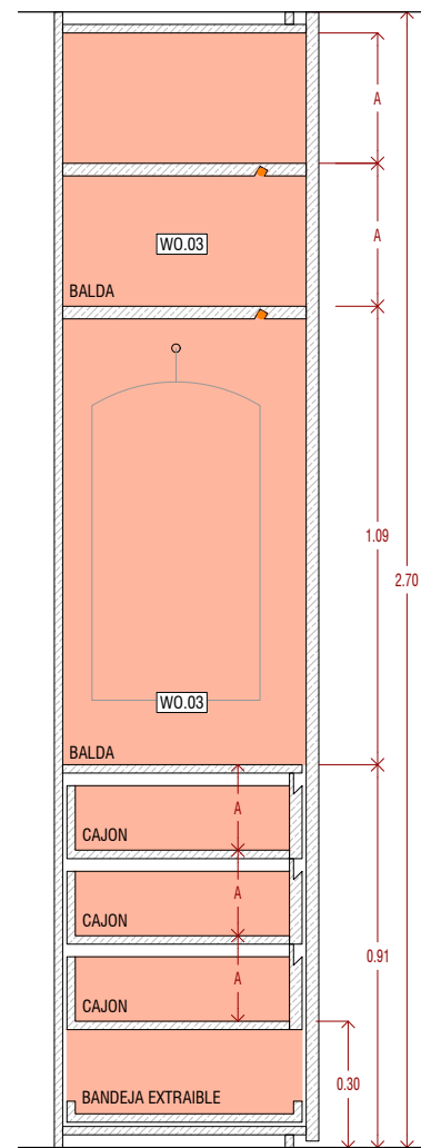
S02
