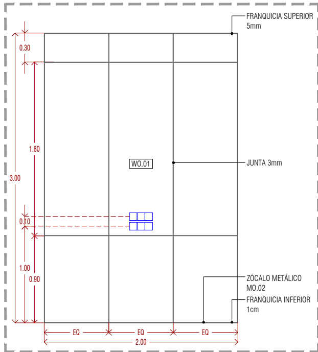
DESPIECE PANEL DORMITORIO SECUNDARIO 01 VER MUEBLE A MEDIDA FF.130
