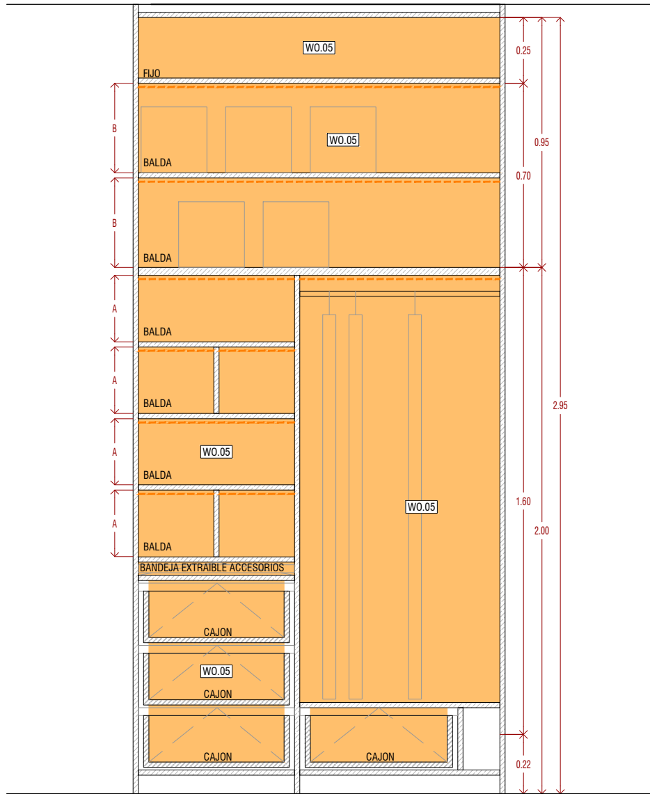
SECCIÓN 03
