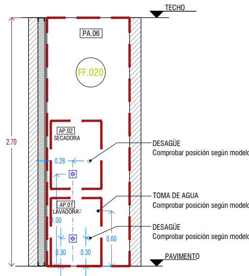
ALZADO 01
