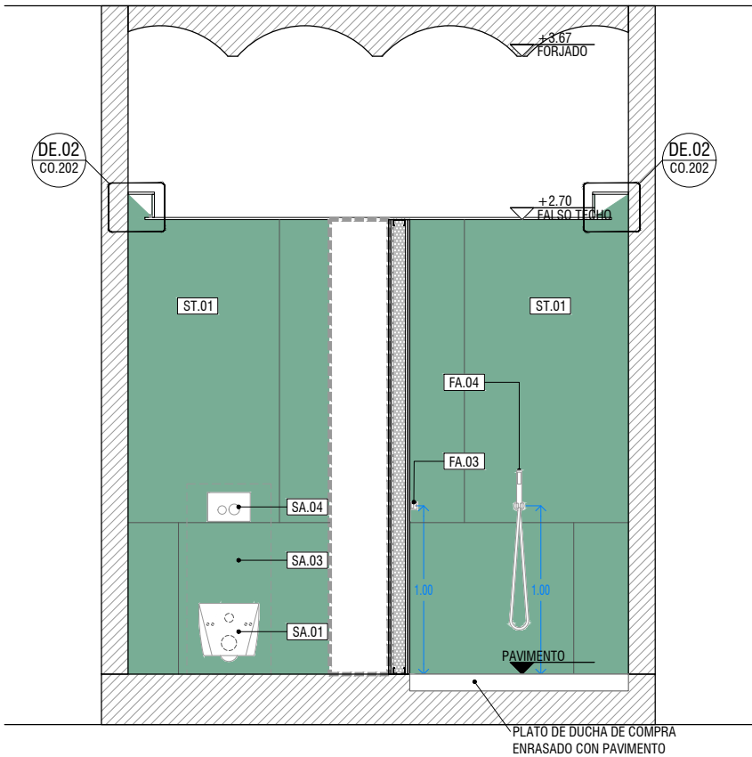
SECCION 04
