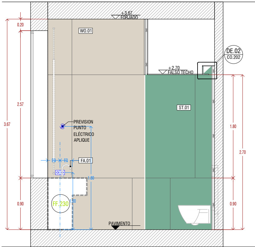
SECCION 02
