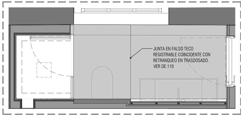
DESPIECE DE TECHO REGISTRABLE. BAÑO SECUNDARIO 01
