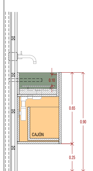
SECCIÓN 02
