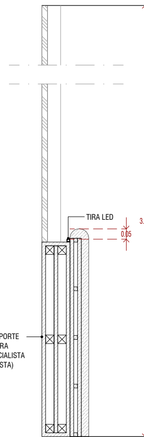
SECCIÓN TRANSVERSAL
