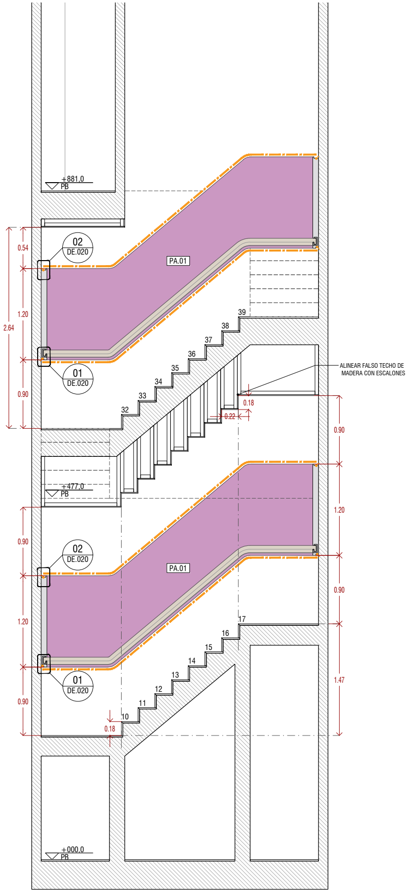
SECCIÓN 03
