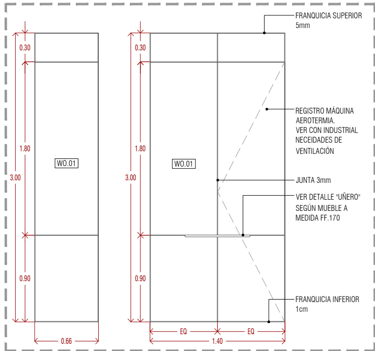
DESPIECE PANEL DORMITORIO SECUNDARIO 02 VER MUEBLE A MEDIDA FF.170
