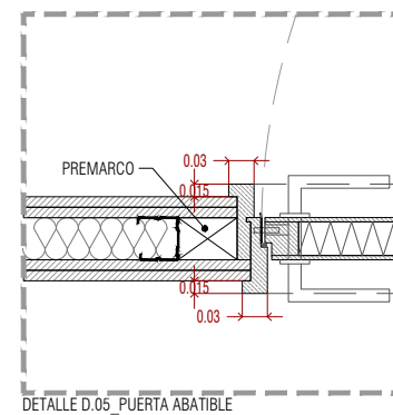
DETALLE D.05 _PUERTA ABATIBLE
