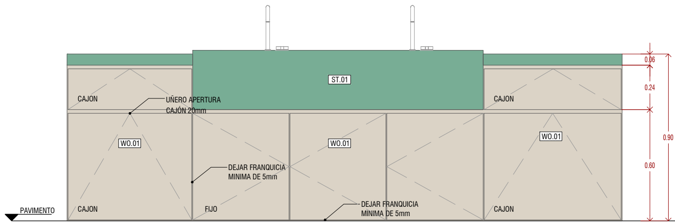
SECCIÓN LONGITUDINAL
