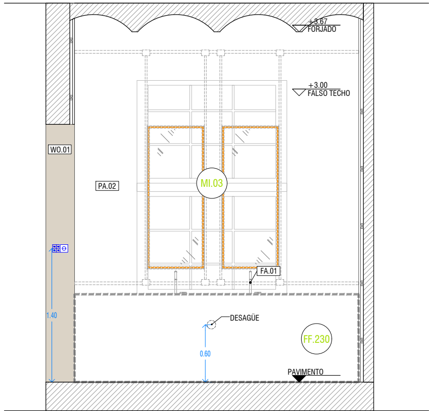
SECCION 01
