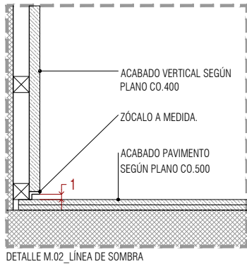
DETALLE M.02 _LÍNEA DE SOMBRA
