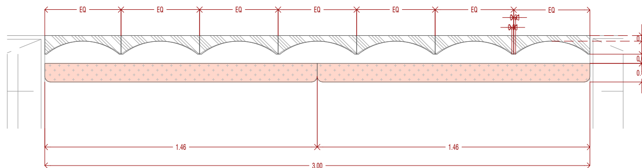
ALZADO
