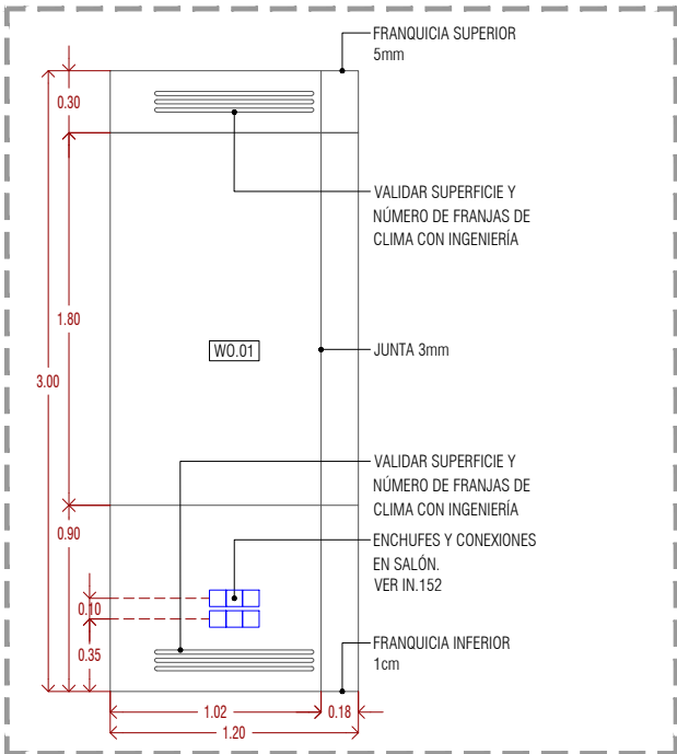
DESPIECE PANEL SALÓN SÍMIL CARPINTERÍA IC.05
