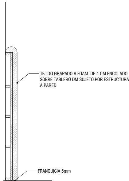
SECCIÓN
