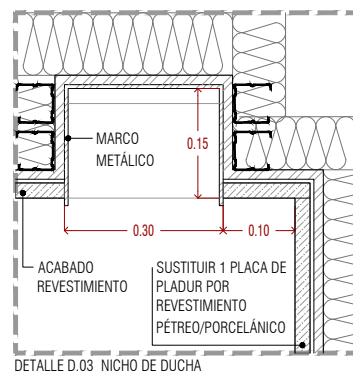
DETALLE D.03 _NICHOS DE DUCHA
