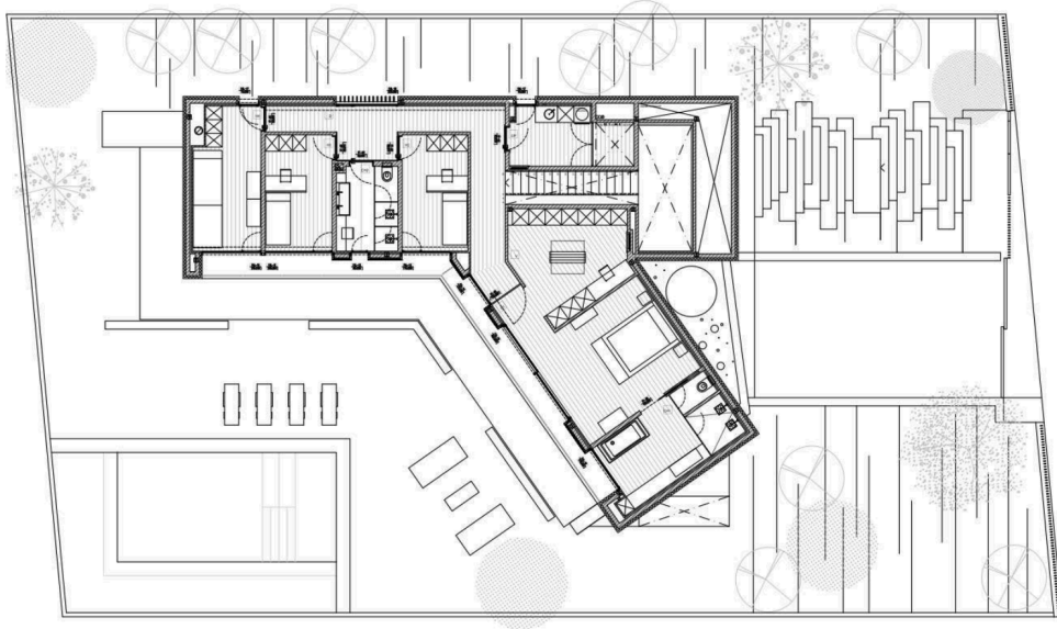
PLANTA PRIMERA FIRST FLOOR
